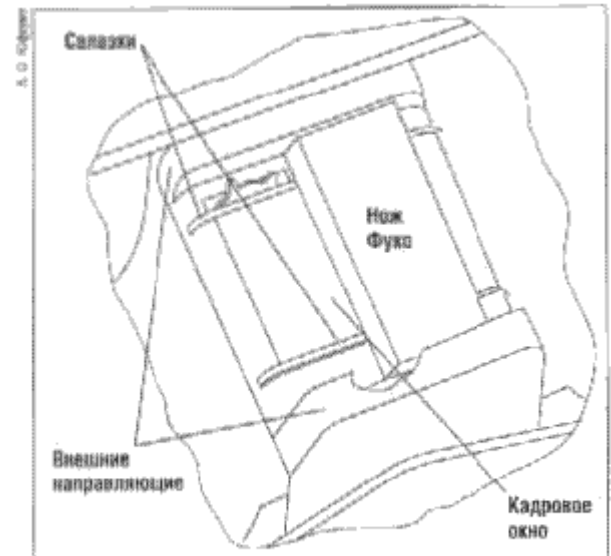
Рис. 1 Нож Фуко устанавливается прямо на слезки между внешними направляющими.
