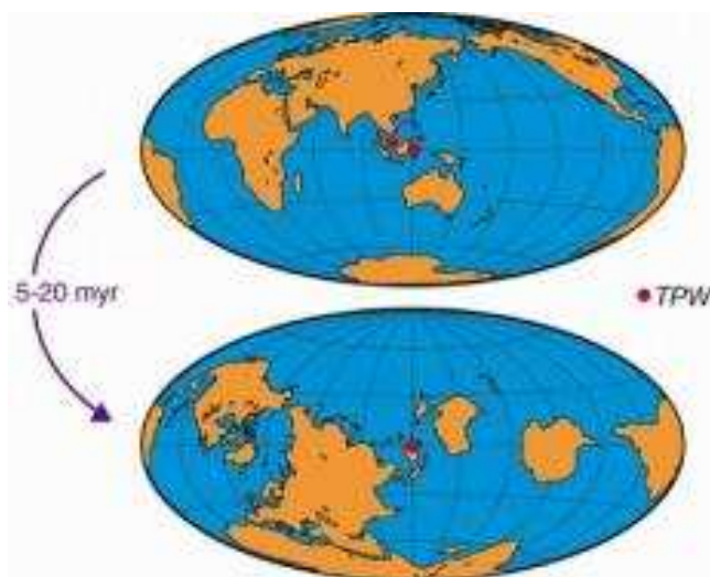
Схема смены земных полюсов в результате смещения континентов. Изображение с сайта http://www.universetoday.com/
