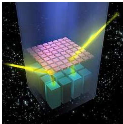
«Интеграл» может фиксировать излучение одновременно от разных источников (рисунок художника). Изображение с сайта http://www.universetoday.com/
